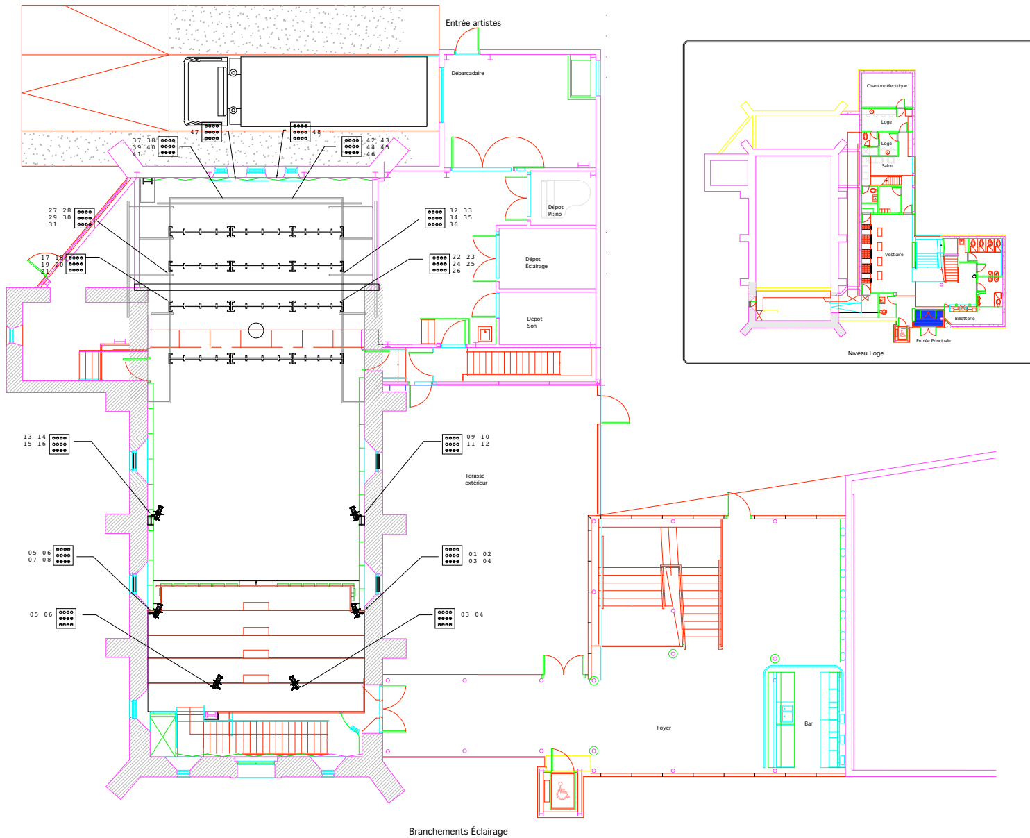
Branchements Éclairage
